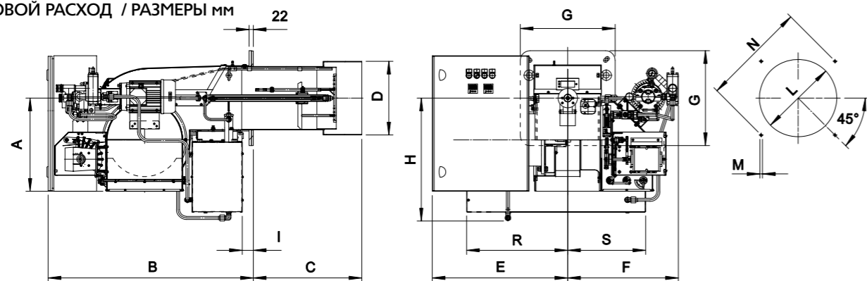
ТЕПЛОВОЙ РАСХОД / РАЗМЕРЫ мм
