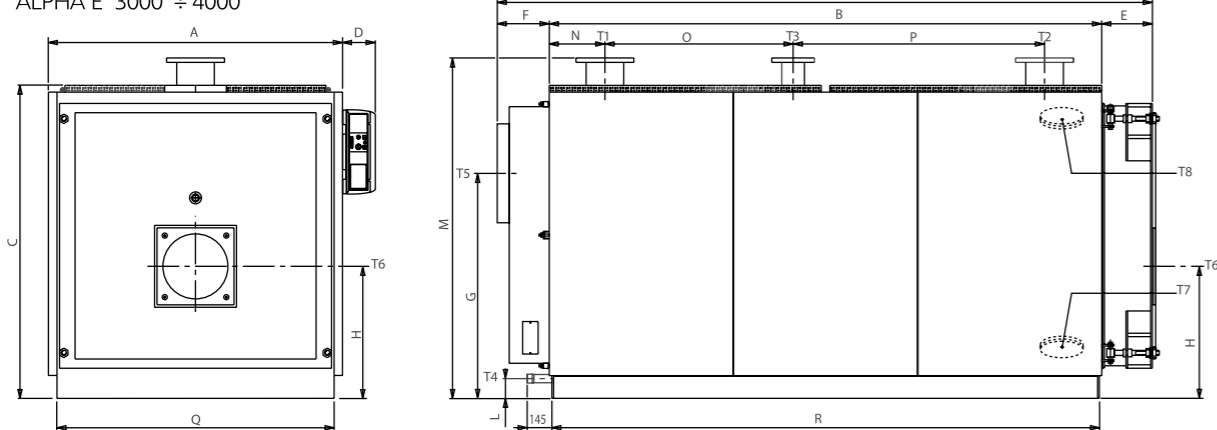
ALPHA E 3000 ÷ 4000
