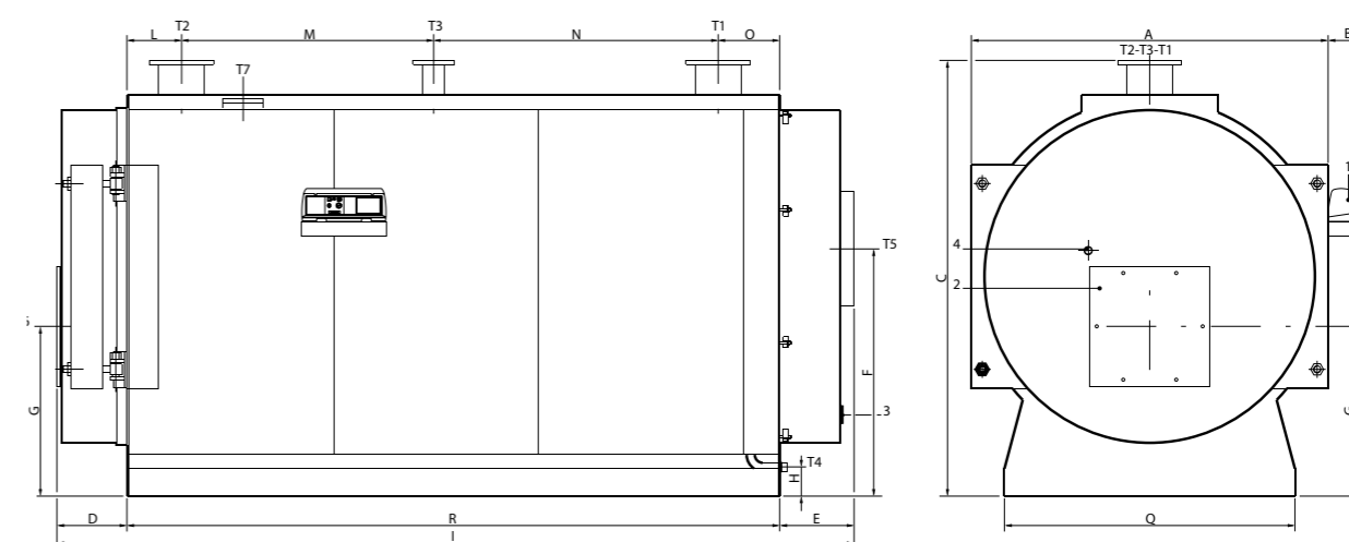
ALPHA E 4500 ÷ 7000
