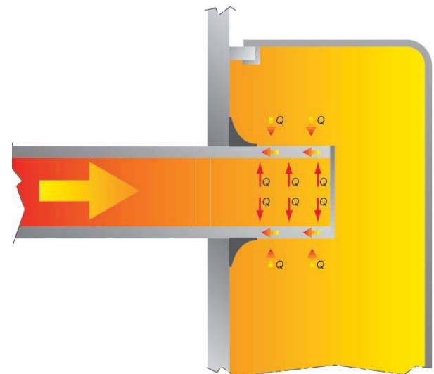
Схема движения дымовых газов УМЕНЬШЕНИЕ ОБРАЗОВАНИЯ КАЛЬЦИЕВЫХ ОТЛОЖЕНИЙ И ШЛАМА
