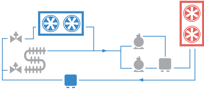
Система непосредственного кипения с каскадной холодильной машиной для охлаждения и заморозки.
