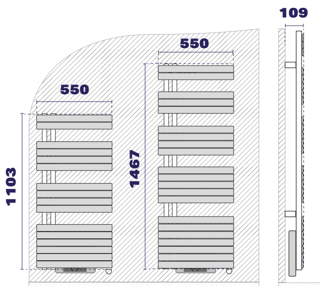
collecteurs verticaux à gauche - soufflant
