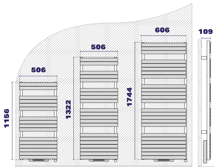
Nantua 3 Éole - soufflant
