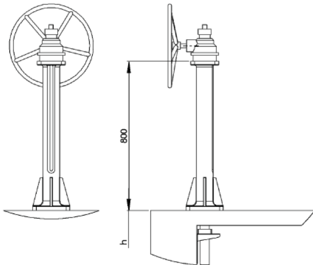
Редуктор и электропривод на прямом пьедестале
