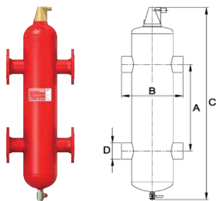
Flexbalance Plus DN = 50 до 125 мм
