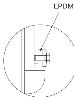
Уплотнение основания
