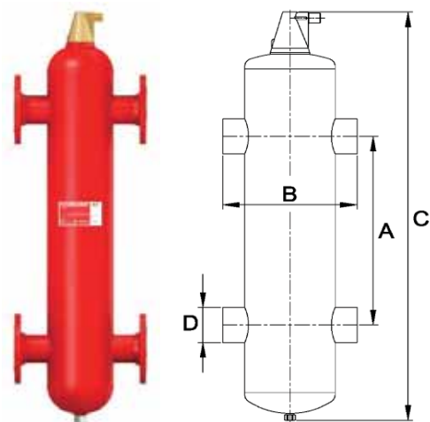
Flexbalance DN = 50 до 125 мм
