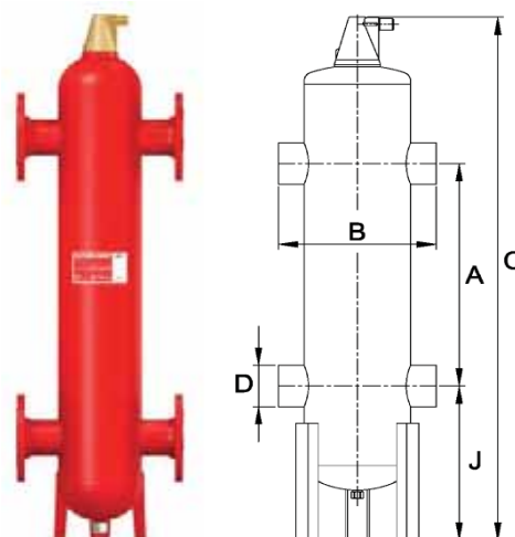
Flexbalance DN = 150 до 400 мм
