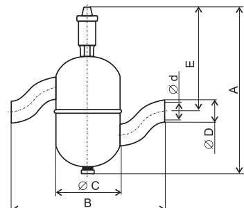
Flexair, присоединение сварка, DN 25–50 мм
