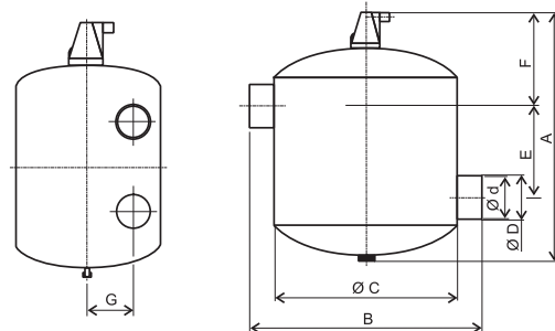
Flexair, присоединение сварка, DN 65–600 мм
