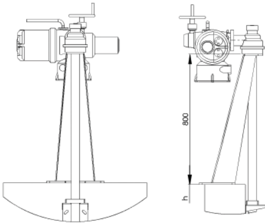
Редуктор с приводом на наклонном пьедестале
