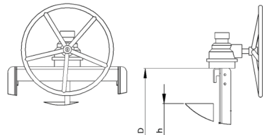
Редуктор на корпусе
