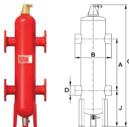
Flexbalance Plus DN = 150 до 400 мм
