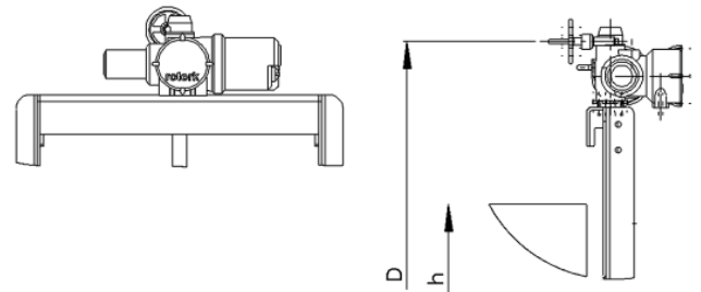
Электропривод на корпусе
