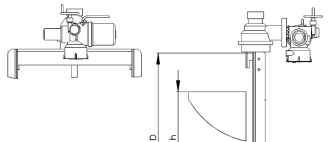
Редуктор и электропривод на корпусе
