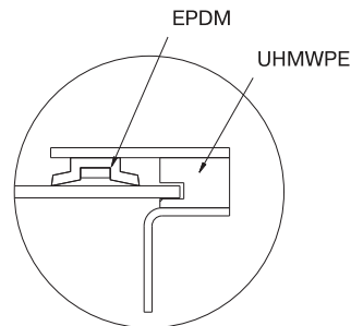
Боковое уплотнение
