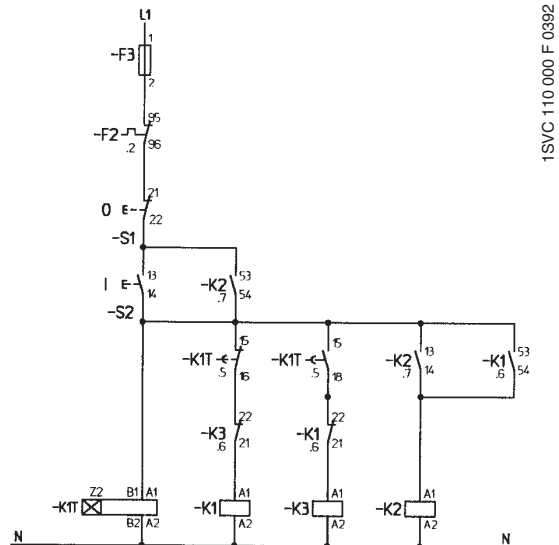
Схема управления
