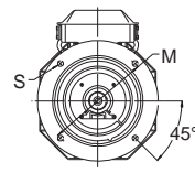
Типоразмеры 90-180
