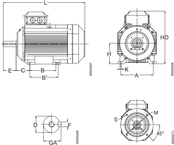
Типоразмеры 71-200
